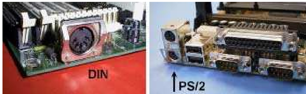
Figura 1.4 Conectores para teclado.
