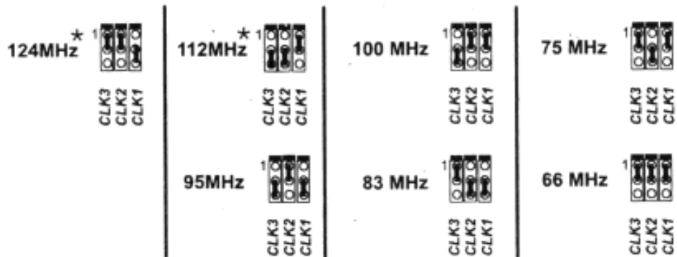
Figura 3.5 Programação de clock externo.
